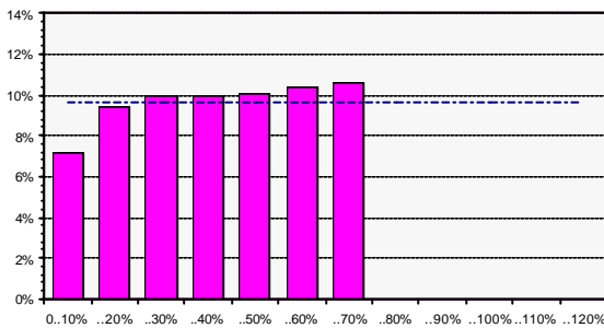
Fig. 7.3.7: Systemwirkungsgrad \eta_{TOT}^* [%] vs. Leistungsbereich PAC/PDC STC
