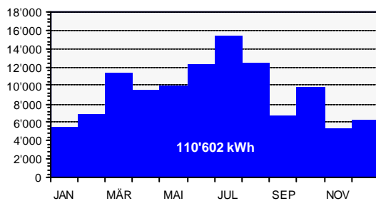
Fig. 15.3.18: Energieerträge [kWh/Mt]
