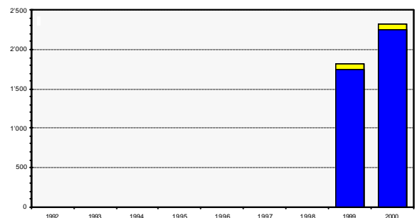
Fig. 11.2.9: Array-Betriebsstunden (blau) und Sonnenstunden (gelb) [%]
