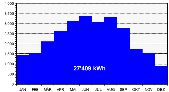
Fig. 11.3.1: Monatliche Energieerträge [kWh/Mt]
