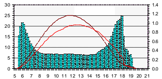
Fig. 15.3.7: Abweichung zwischen Pyranometer- und Referenzzellenmessung in [% des Pyranometerwertes] auf der linken Skala, Yr,h (hellrot) und Yr (dunkelrot) in [kWh/kWp/h] auf der rechten Skala
