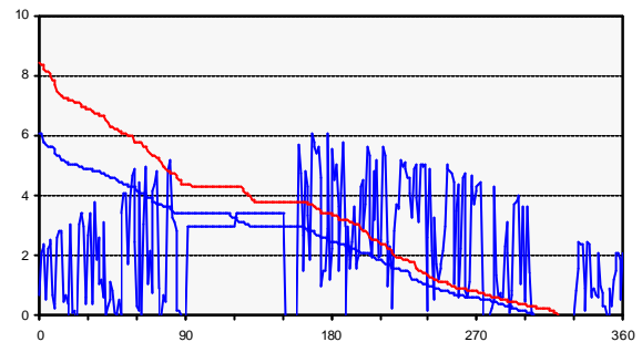
Fig. 11.3.2: Tageswerte Yr (rot) und Yf (blau), chronologisch und geordnet [kWh/kWp/d]
