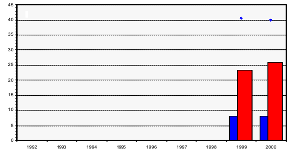
Fig. 11.2.5: Umgebungstemperatur T amb (rot) und gewichtete Generatortemperatur T ag (blau). Als Punkte sind die jeweiligen maximalen 10'-Mittelwerte von T ag aufgetragen.
