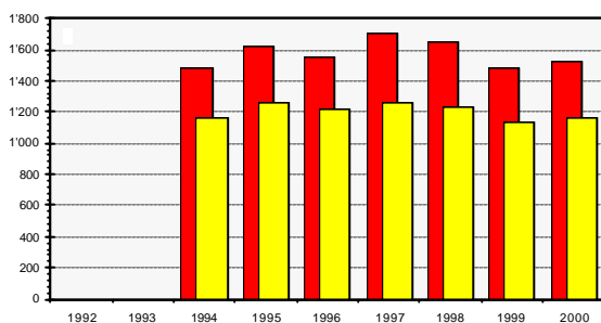
Fig. 8.2.4: Jährliche Globalstrahlung G_{ap} (rot) und G_{hp} (gelb).
