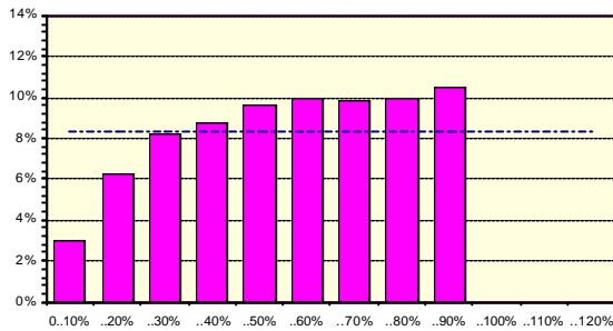
Fig. 5.3.7: Systemwirkungsgrad \eta_{TOT}^* [%] vs. Leistungsbereich PAC/PDC STC
