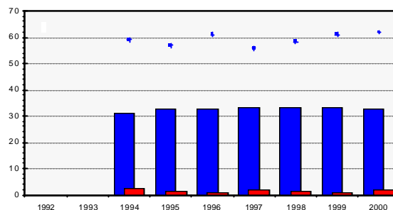
Fig. 8.2.5: Umgebungstemperatur T_{amb} (rot) und gewichtete Generatortemperatur T_{ag} (blau). Als Punkte sind die jeweiligen maximalen 10'-Mittelwerte von T_{ag} aufgetragen.
