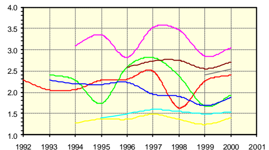
Fig 3.1.3: Jahresertrag Y f [kWh ac /kW p /d]. Anlagen gem. Fig. 3.1.1
