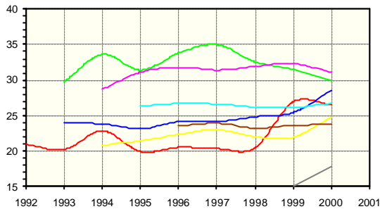
Fig 3.2.5: Modulerwärmung (gewichtete Modultemperatur – Lufttemperatur) [°C]: BAD = rot, FIN = grün, BRU = dunkelblau, STE = gelb, DIS = violett, WIN = hellblau, BUC = braun, EWB = grau
