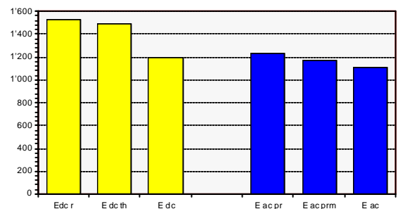
Fig 8.3.3: Jahresarrayertrag E dc (gelb): Referenz (T m =25°C), theoretisch (temperaturkorrigiert) und effektiv (gemessen); Jahresenergie ins Netz E ac (blau): Prognose (Meteonorm), Prognose (witterungs-bereinigt), effektiv (gemessen) [kWh/kWp/a]
