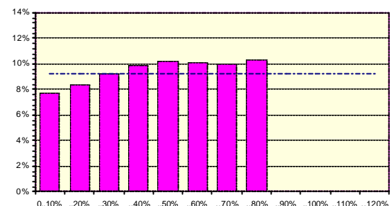
Fig. 6.3.7: Systemwirkungsgrad \eta_{TOT}^* [%] vs. Leistungsbereich PAC/PDC STC
