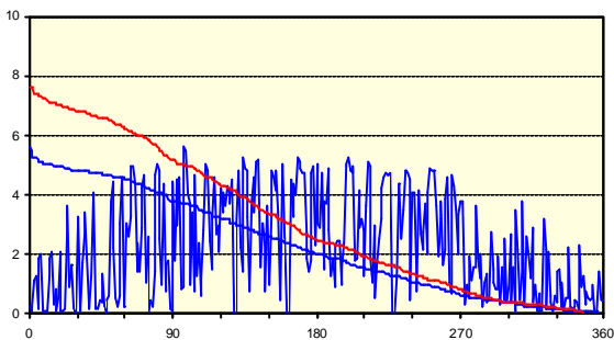
Fig. 4.3.2: Tageswerte Yr (rot) und Yf (blau), chronologisch und geordnet [kWh/kWp/d]
