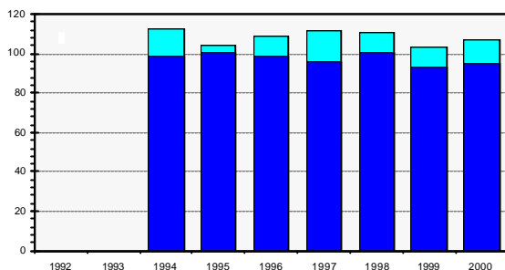
Fig. 8.2.3: Höchste Momentanleistungen in [%] der Nominalleistung (DC, STC). Hellblau: 10'-Mittelwert; dunkelblau: 1h-Mittelwert.
