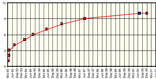
Fig. 7.2.0: Kumulierte Anzahl der Modul-Glasbrüche. Zwar ist das Problem nicht behoben, die Bruchhäufigkeit ist jedoch abnehmend.
