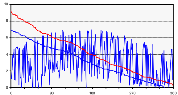
Fig. 8.3.2: Tageswerte Yr (rot) und Yf (blau), chronologisch und geordnet [kWh/kWp/d]
