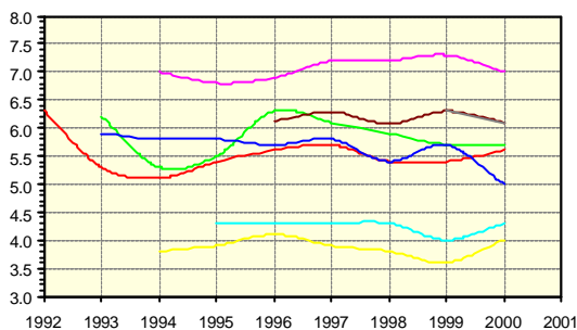
Fig 3.1.2: Höchste Tageserträge [kWh ac /kW p /d]. Anlagen gem. Fig. 3.1.1
