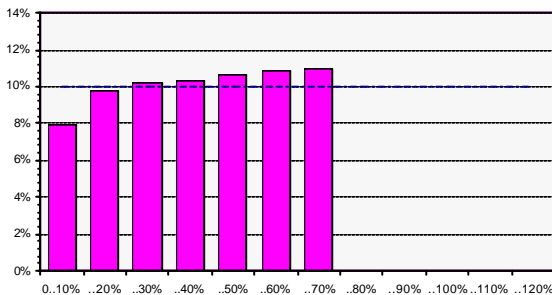
Fig. 9.3.7: Systemwirkungsgrad \eta_{TOT}^* [%] vs. Leistungsbereich PAC/PDC STC
