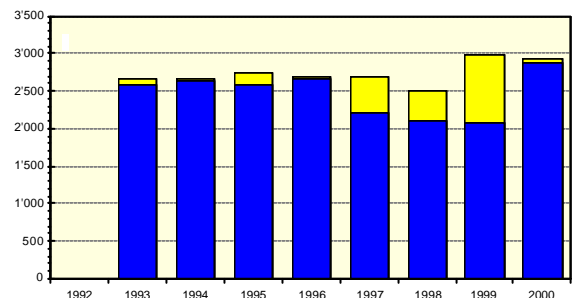
Fig. 6.2.7: Array-Betriebsstunden (blau) und Sonnenstunden (gelb) [%]
