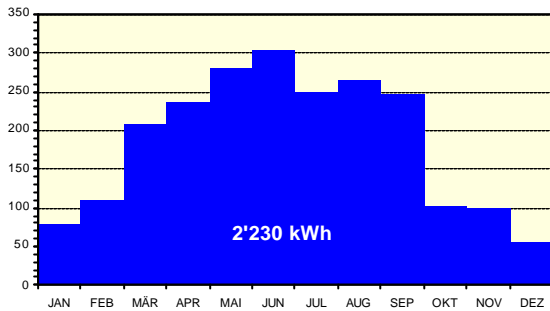
Fig. 4.3.1: Monatliche Energieerträge [kWh/Mt]
