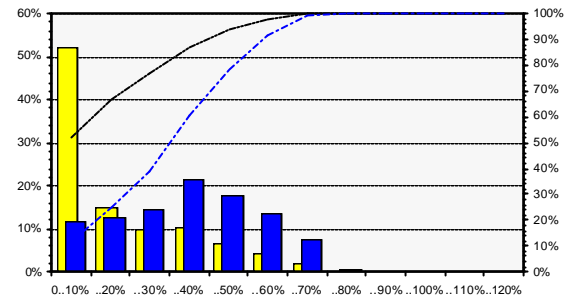
Fig. 9.3.4: Häufigkeit der Betriebsstunden (gelb) und des Energieertrages (blau) vs. Leistungsbereich PAC/PDC STC. Linien: Summenhäufigkeit
