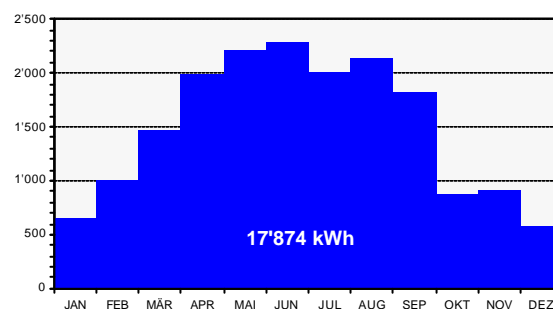
Fig. 10.3.1: Monatliche Energieerträge [kWh/Mt]
