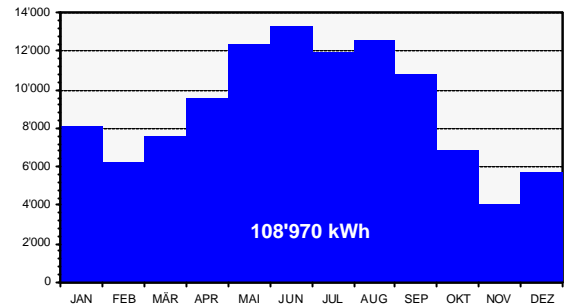
Fig. 8.3.1: Monatliche Energieerträge [kWh/Mt]
