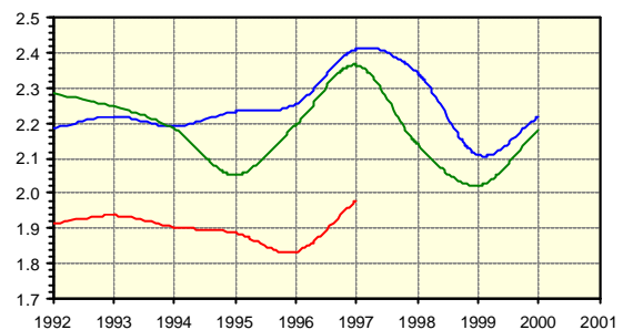
Fig 3.1.4: Jahresertrag Y f [kWh ac /kW p /d] der Messkampagnen des 1000-Dächer-Programms (rot, wurde Ende 1997 abgeschlossen), der VSE-PV-Statistik (blau) und der 1-MW-Solarkette der NOK (grün)
