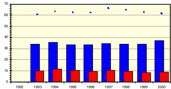
Fig. 6.2.5: Umgebungstemperatur T_{amb} (rot) und gewichtete Generatortemperatur T_{ag} (blau). Als Punkte sind die jeweiligen maximalen 10'-Mittelwerte von T_{ag} aufgetragen.
