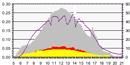
Fig. 15.3.6: L_s (gelb), L_{CT} (rot) und L_{CM} in [kWh/kWp/h] auf der linken Skala, gewichtete Modultemperatur in [°C] auf der rechten Skala
