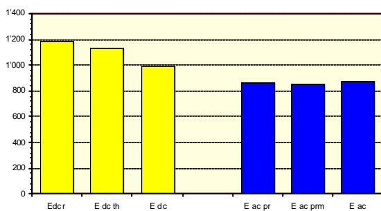
Fig 4.3.3: Jahresarrayertrag E dc (gelb): Referenz ( T_m=25^\circ\text{C} ), theoretisch (temperaturkorrigiert) und effektiv (gemessen); Jahresenergie ins Netz E ac (blau): Prognose (Meteonorm), Prognose (witterungsbereinigt), effektiv (gemessen) [kWh/kWp/a]
