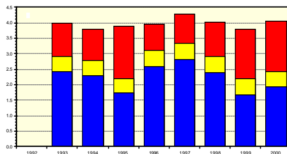
Fig. 5.2.1: Spezifische Jahreserträge Yr (rot), Ya (gelb) und Yf (blau) [kWh/kWp/d]
