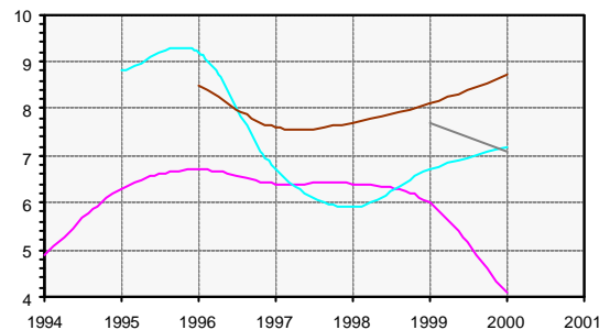
Fig. 12.2.1: Mittlere jährliche Differenz zwischen Pyranometer und c-Si-Referenzzellen in [% Pyranometer]: DIS = violett, WIN = hellblau, BUC = braun.
