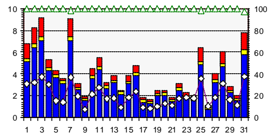
Fig. 15.3.8: Spezifische Erträge Yr, Ya (gelb) und Yf (blau) in [kWh/kWp/d], auf der linken Skala, gewichtete Modultemperatur und Systemverfügbarkeit auf der rechten Skala
