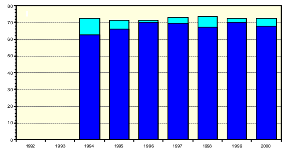
Fig. 7.2.3: Höchste Momentanleistungen in [%] der Nominalleistung (DC, STC). Hellblau: 10'-Mittelwert; dunkelblau: 1h-Mittelwert.
