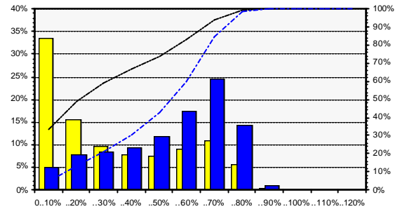
Fig. 10.3.4: Häufigkeit der Betriebsstunden (gelb) und des Energieertrages (blau) vs. Leistungsbereich PAC/PDC STC. Linien: Summenhäufigkeit
