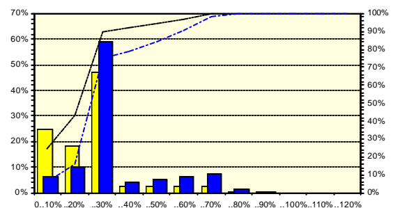
Fig. 6.3.4: Häufigkeit der Betriebsstunden (gelb) und des Energieertrages (blau) vs. Leistungsbereich PAC/PDC STC. Linien: Summenhäufigkeit
