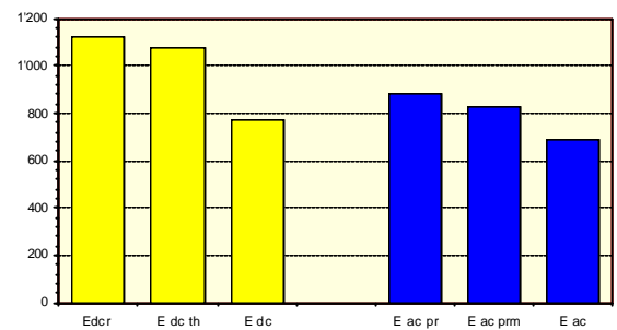
Fig 6.3.3: Jahresarrayertrag E dc (gelb): Referenz (T m =25°C), theoretisch (temperaturkorrigiert) und effektiv (gemessen); Jahresenergie ins Netz E ac (blau): Prognose (Meteonorm), Prognose (witterungs-bereinigt), effektiv (gemessen) [kWh/kWp/a]
