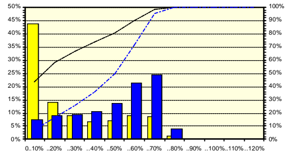
Fig. 4.3.4: Häufigkeit der Betriebsstunden (gelb) und des Energieertrages (blau) vs. Leistungsbereich PAC/PDC STC. Linien: Summenhäufigkeit
