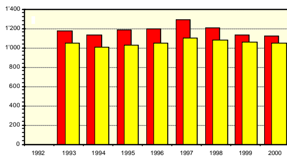
Fig. 6.2.4: Jährliche Globalstrahlung G_{ap} (rot) und G_{hp} (gelb).
