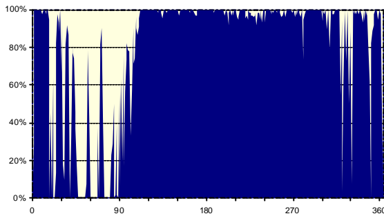
Fig. 5.3.8: Verfügbarkeit der Photovoltaik-Anlage
