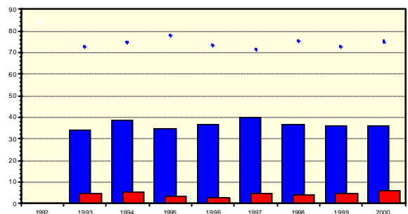
Fig. 5.2.5: Umgebungstemperatur T amb (rot) und gewichtete Generatortemperatur T ag (blau). Als Punkte sind die jeweiligen maximalen 10'-Mittelwerte von T ag aufgetragen.
