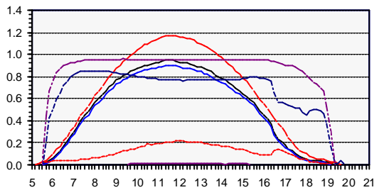
Fig. 15.3.4: Yr (rot, ausgezogen), Ya (schwarz, ausgezogen), Yf (blau, ausgezogen), L_{CM} (rot, gestrichelt), L_{CT} (violett, strich-punktiert), PR (dunkelblau, ausgezogen), \eta_{Inv} (violett, strich-punktiert)
